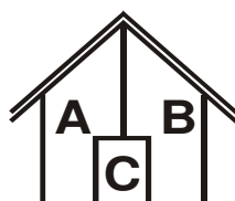
3. Podział na 2 strefy załączenie A lub B. Strefa C załącza się automatycznie, kiedy załączone A+B
