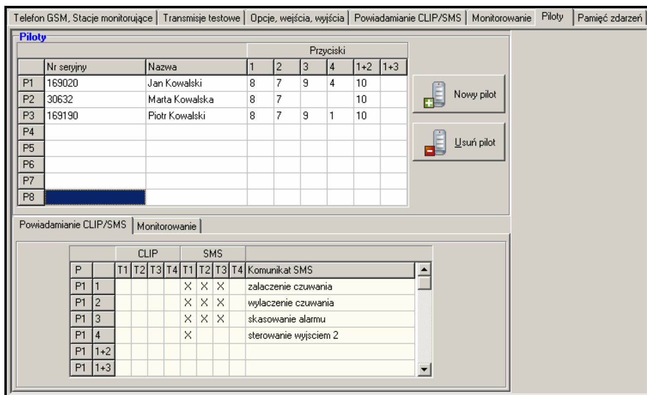
Rys. 15. Zakładka „Piloty”.
