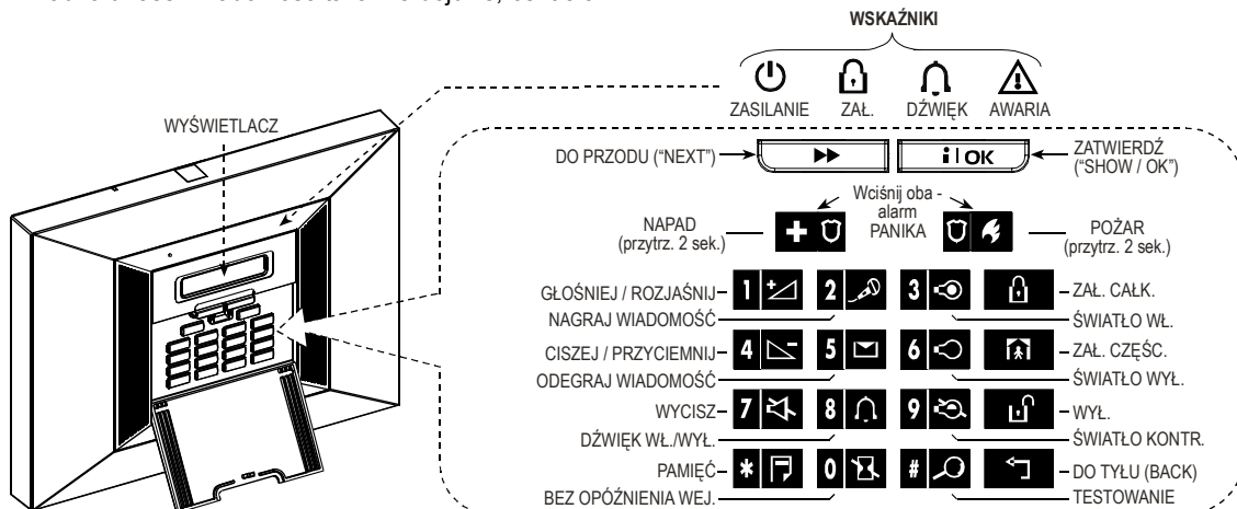
Rys.3. Klawisze i wskaźniki
