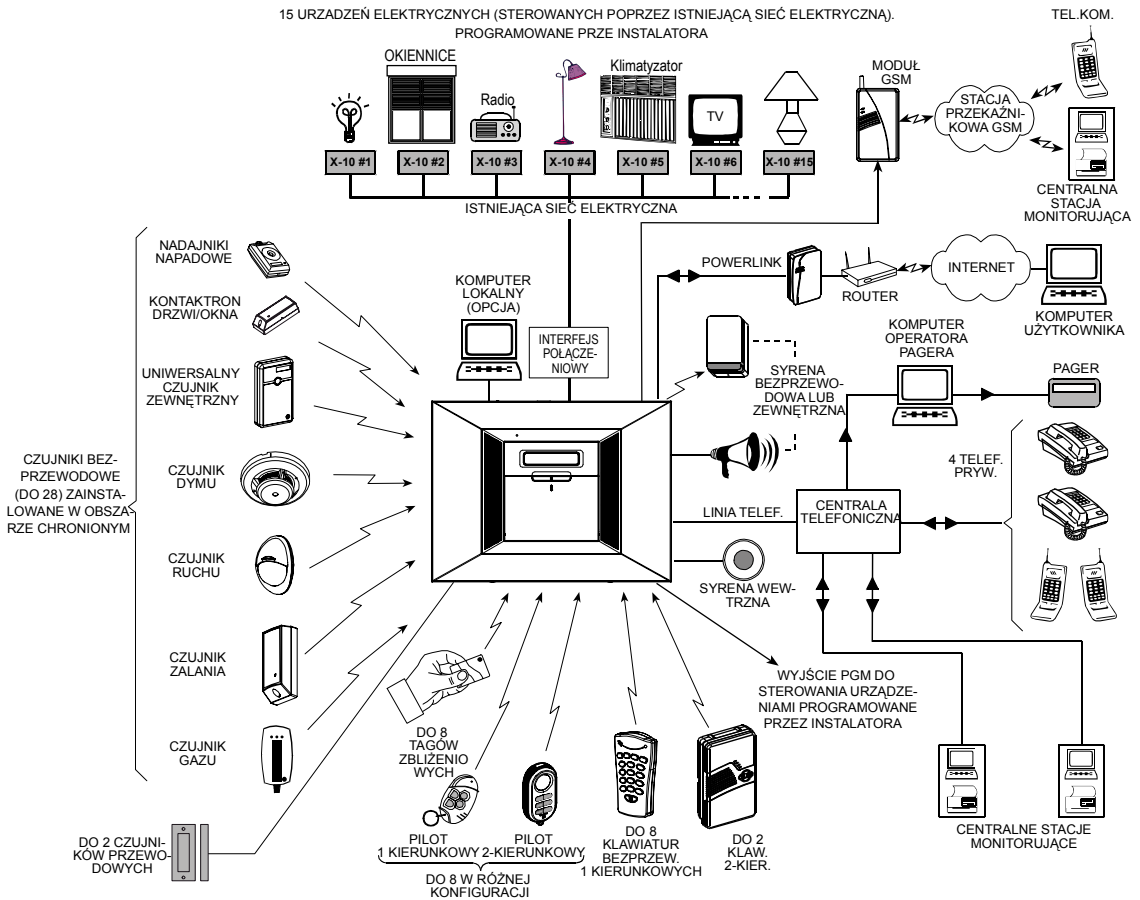
Rys 2. Typowa konfiguracja systemu
